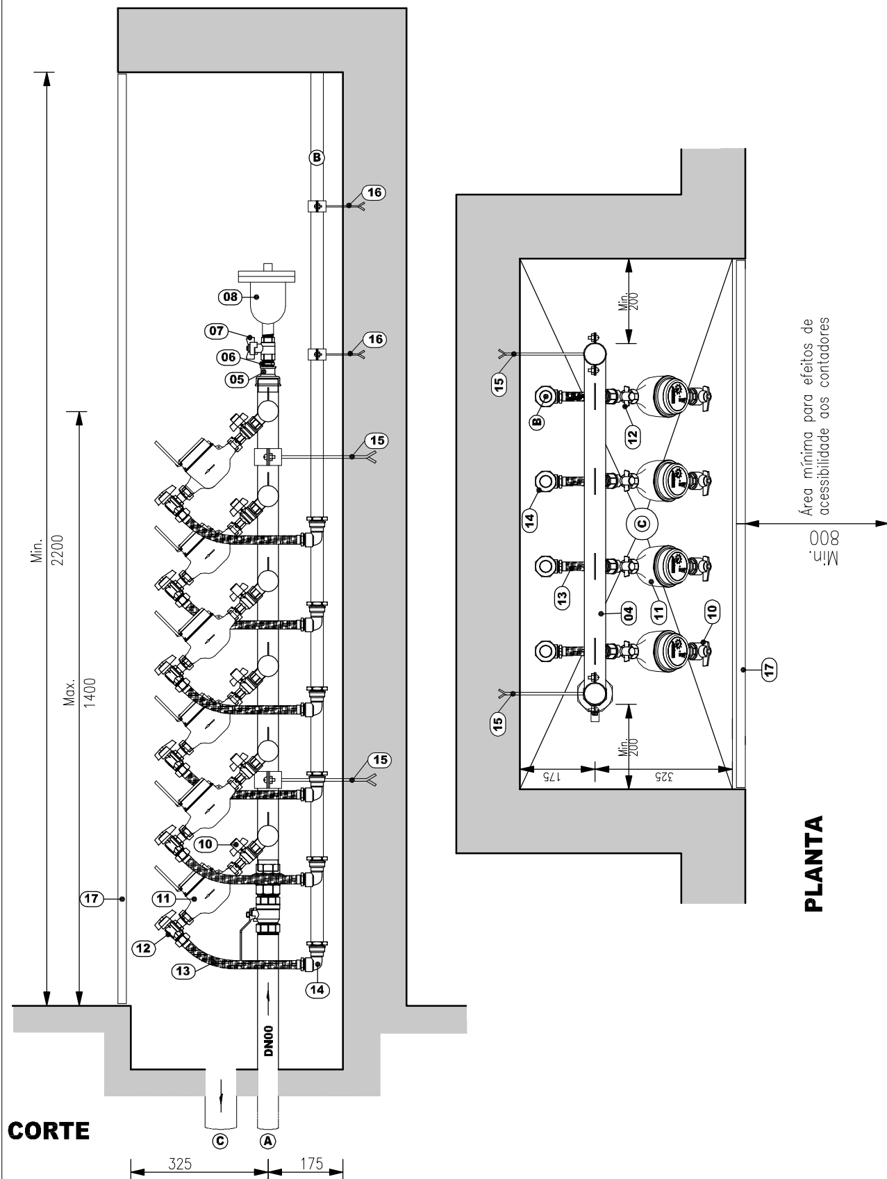
Fig. 1. - Esquema de montagem de bateria - Planta e Corte (Medidas em milímetros)
