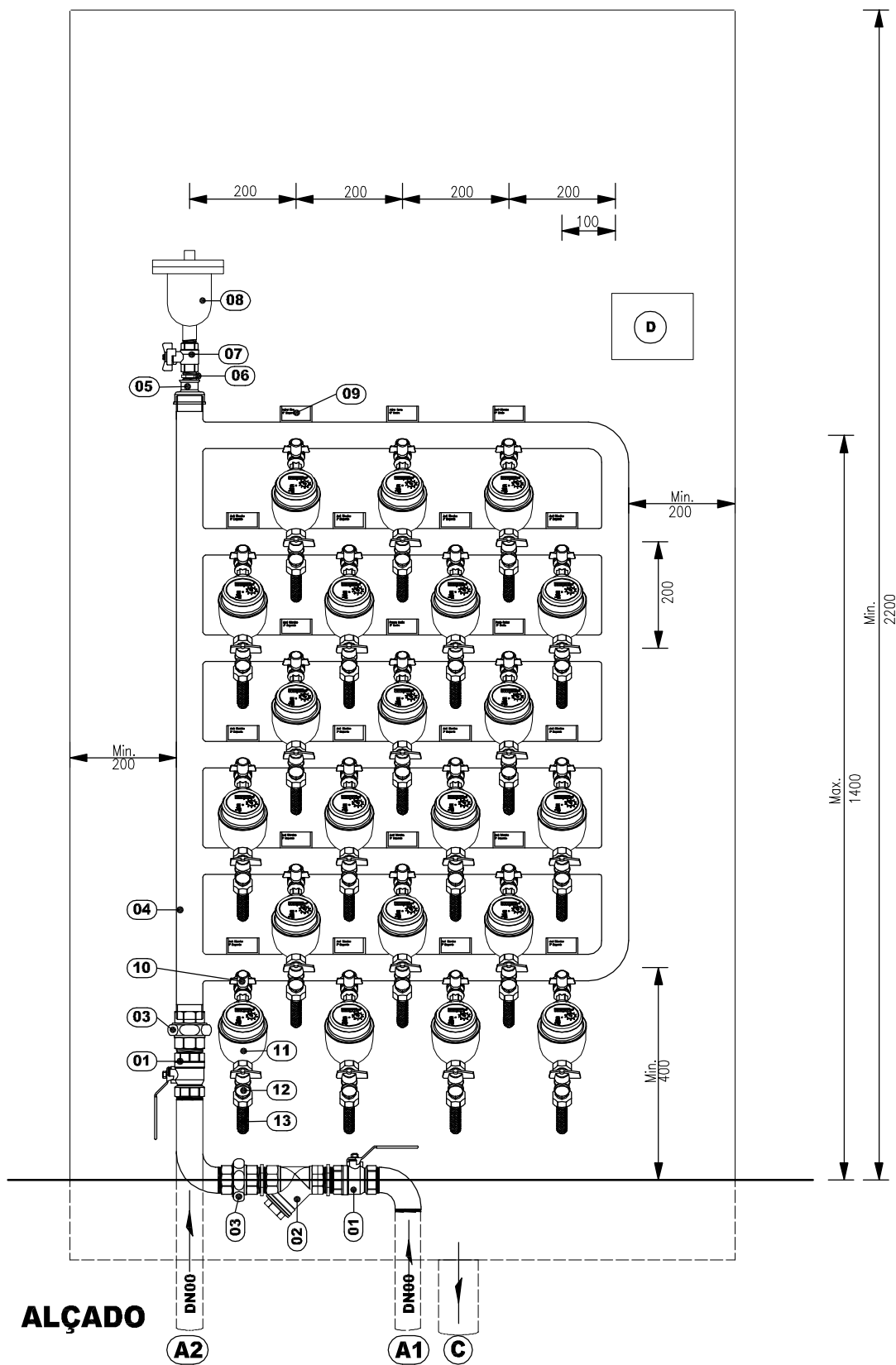
Fig. 1. – Esquema de montagem de bateria – Alçado Principal Medidas em milímetros
